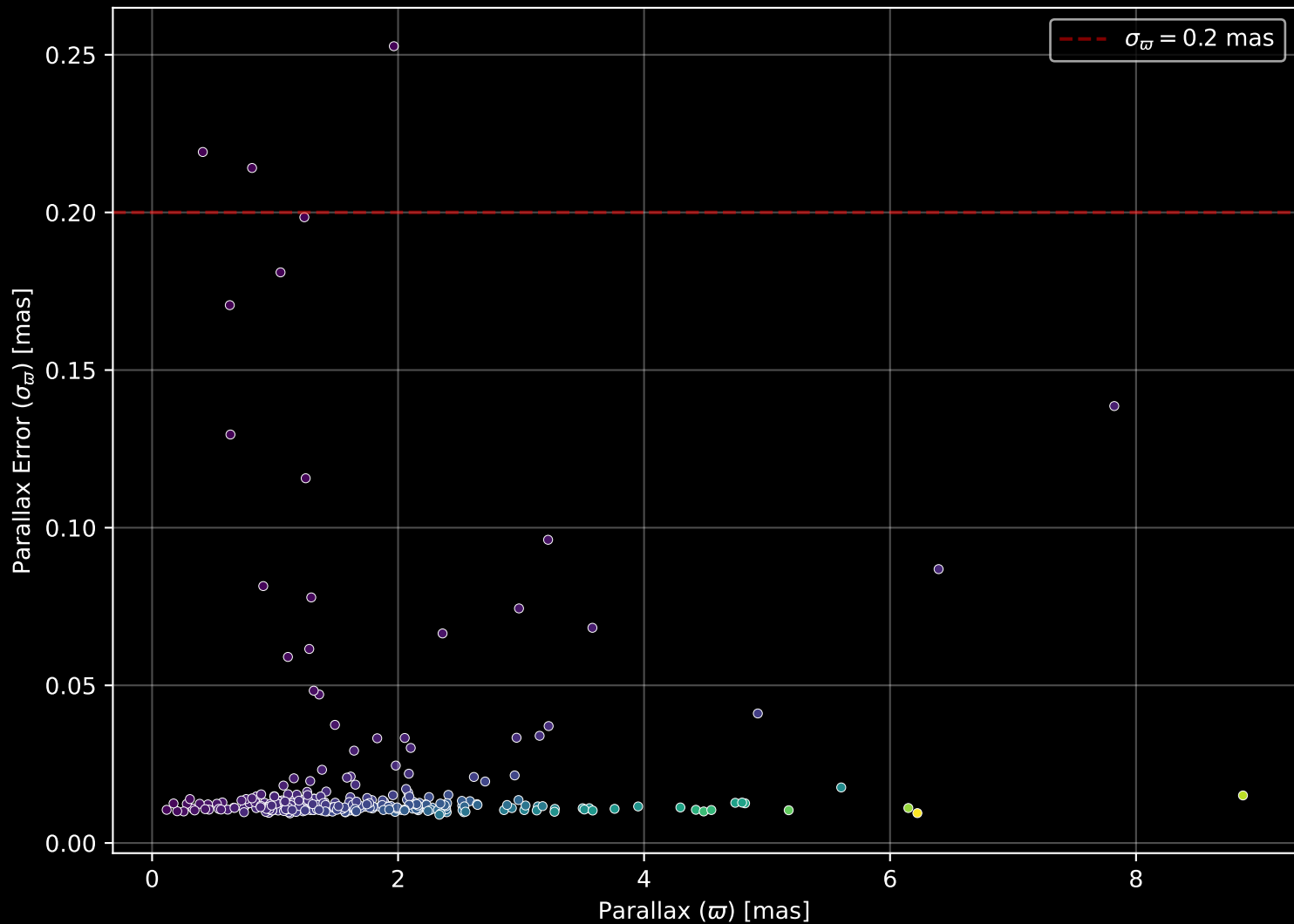
GALAH DR4 Field: [681] Parallax Quality (n= 276)
