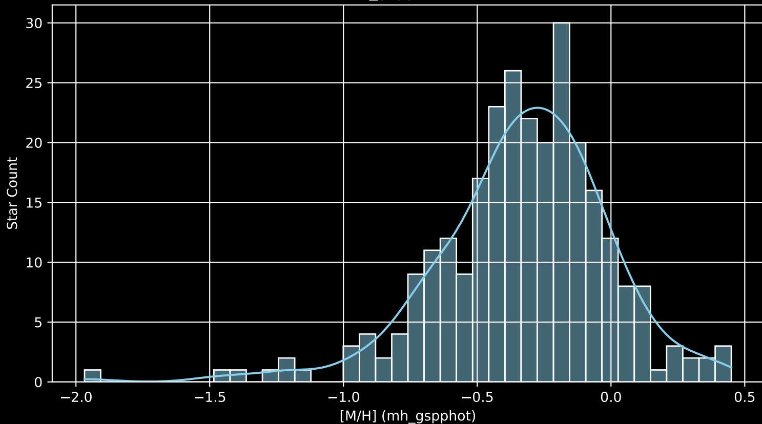
GALAH DR4 Field: [681] [M/H] (mh_gspphot) (n= 274)
