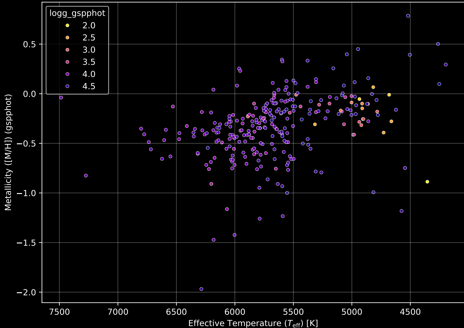
GALAH DR4 Field: [681] Stellar Population Parameters (n= 276)
